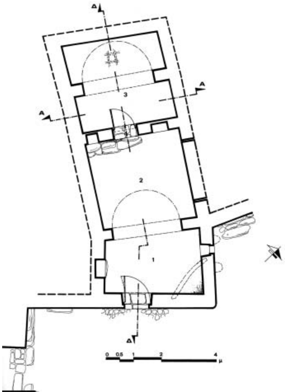
Εκ. 16. Νοφαλιάς: σπίτι του Γραμματικάκη, κάτοψη. 1. πόρτεγο, 2. κάμερα, 3. α-χειρώνας.
