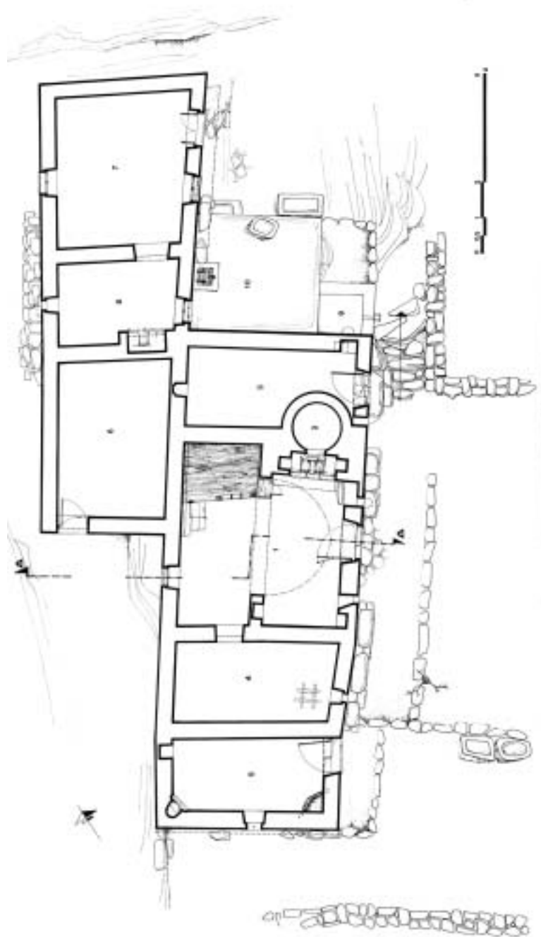
Εικ. 33. Νοφαλιάς: σπίτι του Δεσποτογιόργη, κάτοψη. 1. σπίτι, 2. φούρνος, 3. αργαστηρόσπιτο, 4. αχειρώνας, 5. αχίρι, 6. μάντρα, 7. οντάς, 8. κουζίνα του οντά, 9. πατητήρι, 10. δολωτή στέρνα.
