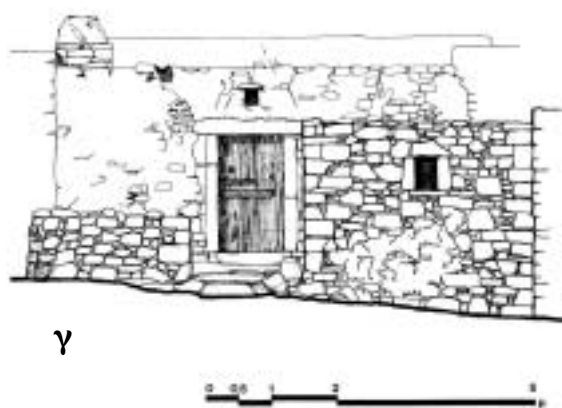
Εικ. 28. Νοφαλιάς: σπίτι του Καρμαλίγκο. α. τομή Α-Α, β. τομή Δ-Δ, γ. πρόσοψη.
