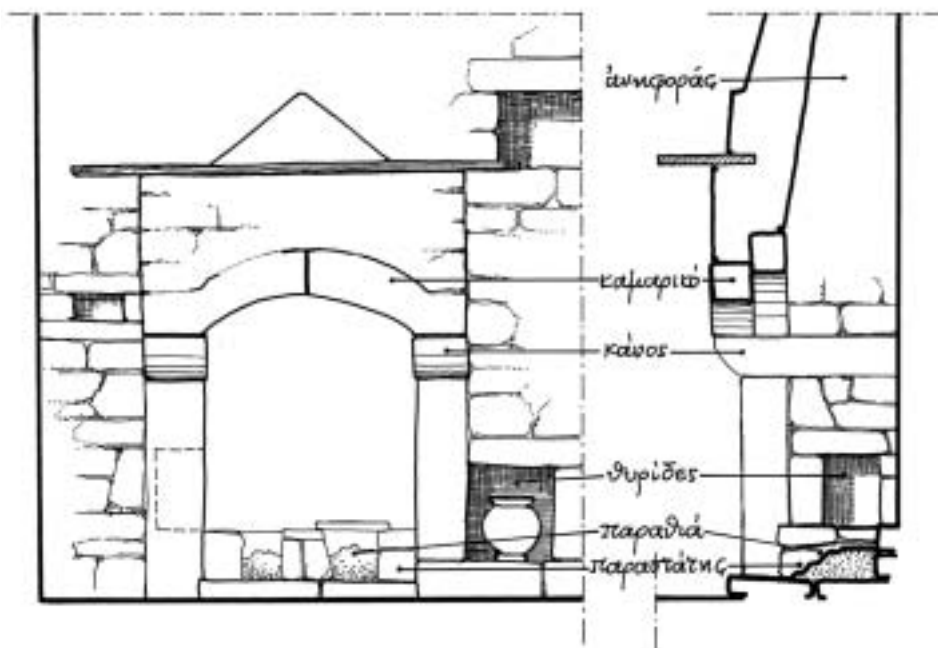
Εικ. 9. Σκαρίφημα χωνευτού τζακιού με κάνους: όψη και τομή.
