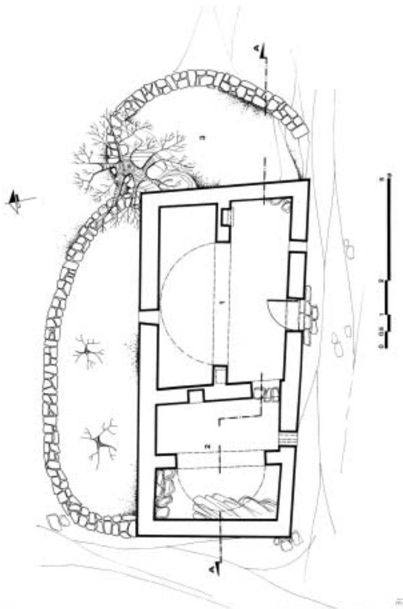
Εικ. 31. Νοφαλίς: το «Μαναστηρικό», κάτοψη. 1. σπίτι, 2. αχειρώνας, 3. υπαίθρια μάντρα.
