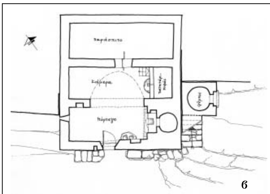
Εικ. 6. Πλατυμέτωπα καμαρόσπιτα – ενδεικτικές κατόψεις. α. Τσολομανόλη, β. Πραξίας (σκαριφήματα).
