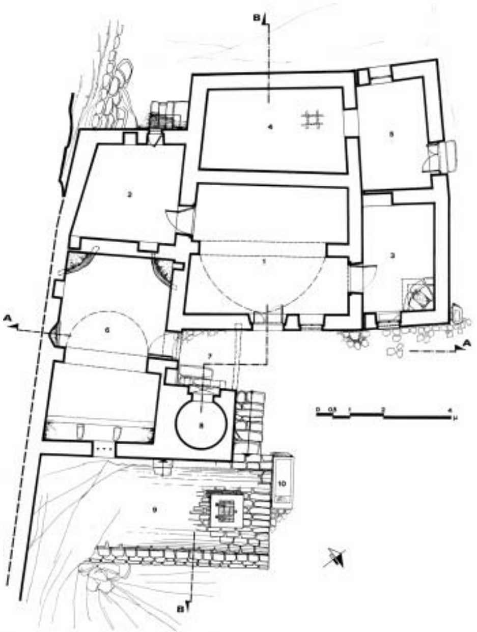
Εικ. 35. Νοφαλιάς: σπίτι του Αριστεΐδη, κάτοψη. 1. σπίτι, 2. κάμερα (υπνοδωμάτιο), 3. κουζίνα, 4. αχειρώνας, 5. αποθήκη, 6. αχίρι, 7. φουρνόσπιτο, 8. φούρνος, 9. δολωτή στέρνα, 10. πλυσταριό.
